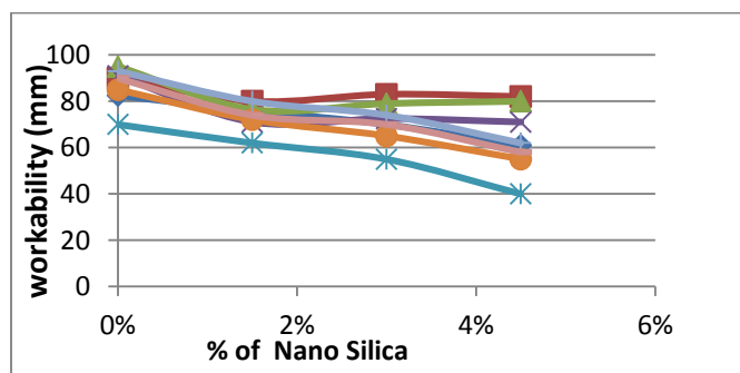
Fig :Workability Test
